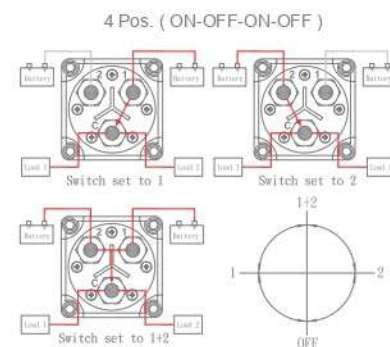
700.12.01.C301121 4 Posiciones (OFF-BAT1-AMBOS-BATERÍA 2)
