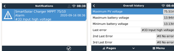
Un dispositivo GX mostrando una notificación de alarma y errores históricos.
