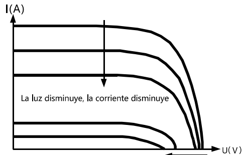
Figure 1-3 Relación entre las características de salida del panel solar y la luz
