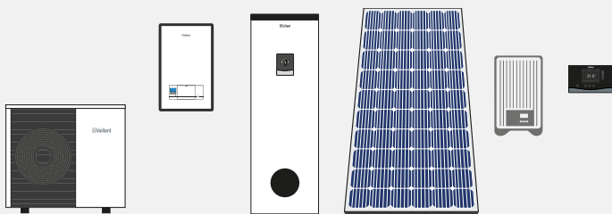
aroTHERM plus con módulo hidráulico VWZ MEH 97, uniTOWER plus VIH RW, módulo fotovoltaico e inversor auroPOWER y control sensoCOMFORT
