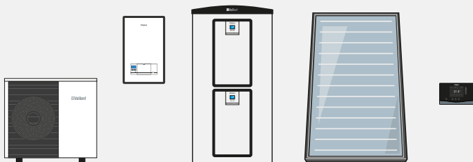
aroTHERM plus con módulo hidráulico VWZ MEH 97, depósito multifunción allSTOR exclusive, captador solar auroTHERM plus y control sensoCOMFORT
