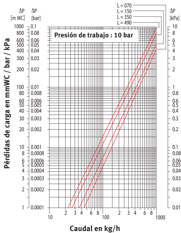
PÉRDIDA DE CARGA TIPO 15
