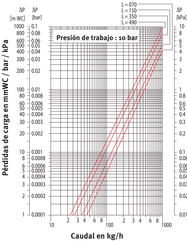
PÉRDIDA DE CARGA TIPO 10
