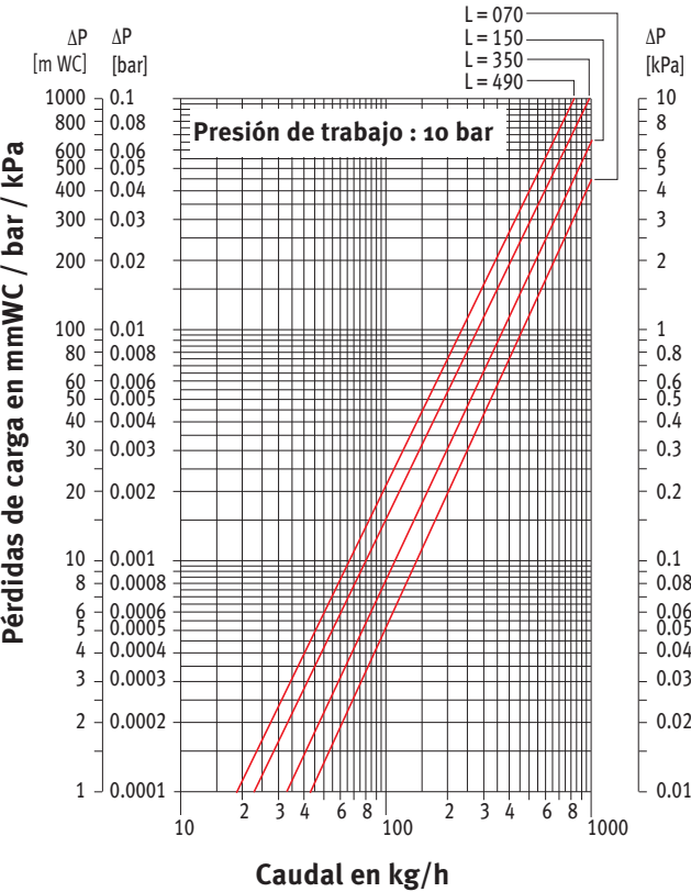
PÉRDIDA DE CARGA TIPO 04 CONEXIONES OPUESTAS
