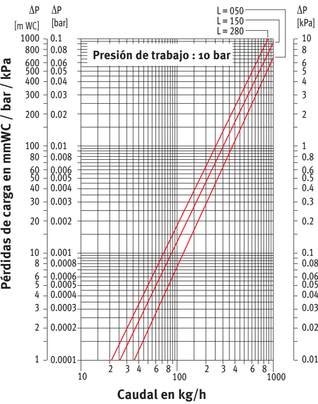
PÉRDIDA DE CARGA TIPO 16
