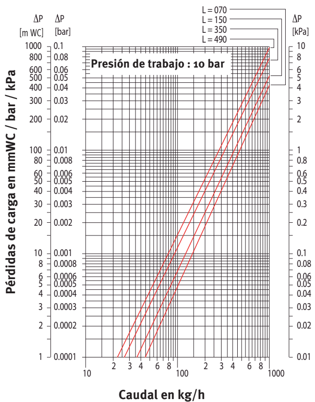
PÉRDIDA DE CARGA TIPO 10
