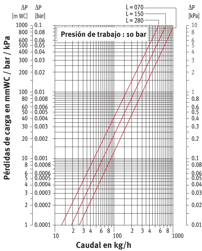
PÉRDIDA DE CARGA TIPO 11
