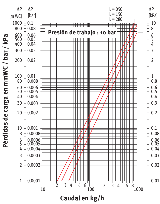
PÉRDIDA DE CARGA TIPO 11
