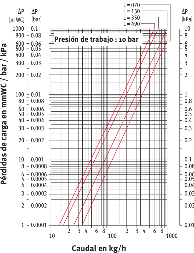
PÉRDIDA DE CARGA TIPO 09
