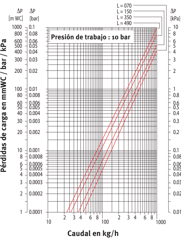
PÉRDIDA DE CARGA TIPO 15
