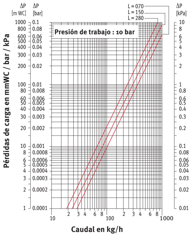
PÉRDIDA DE CARGA TIPO 10
