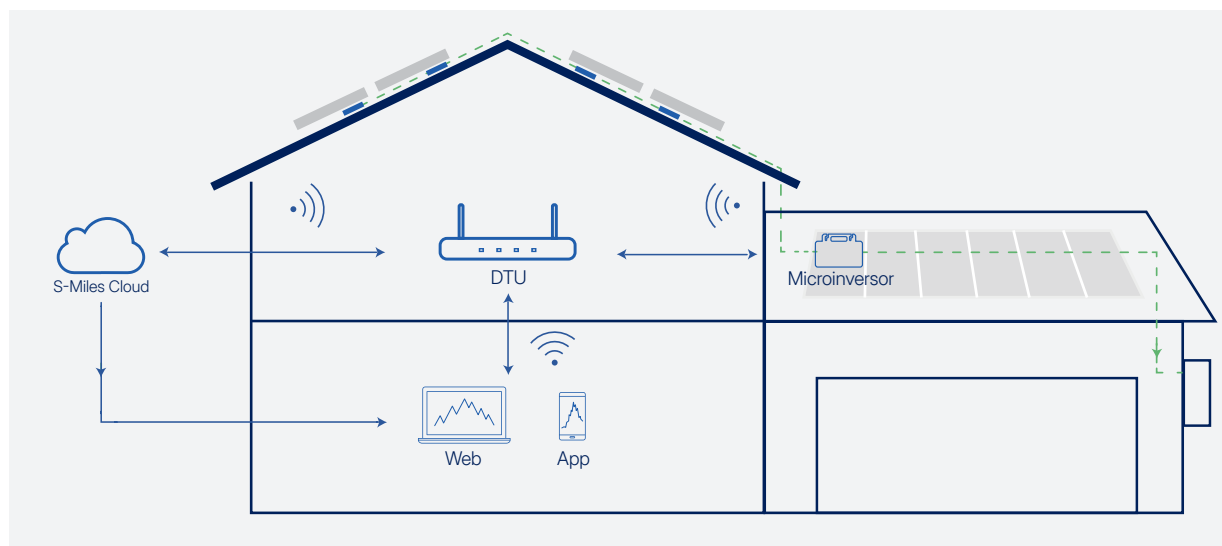
Figura 1-2 Diagrama del sistema de microinversores de la serie HMS-500-1T
