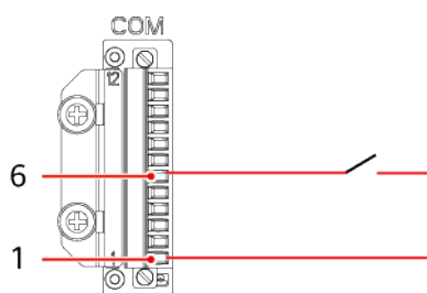
Figura F-1 Conexión de los cables a un interruptor de apagado rápido
