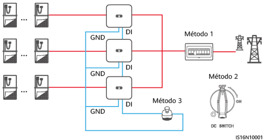
Figura F-2 Métodos de activación de un apagado rápido
