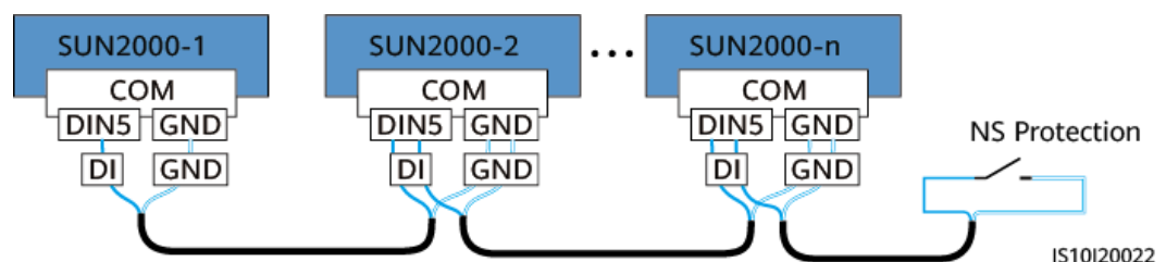
Figura G-1 Conexión de los inversores conectados en cascada al interruptor de protección de NS
