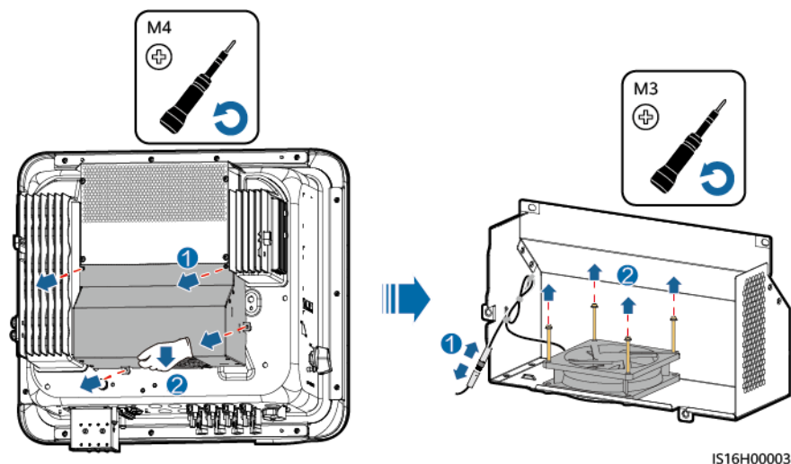
Figura 8-1 Desinstalación del ventilador defectuoso
