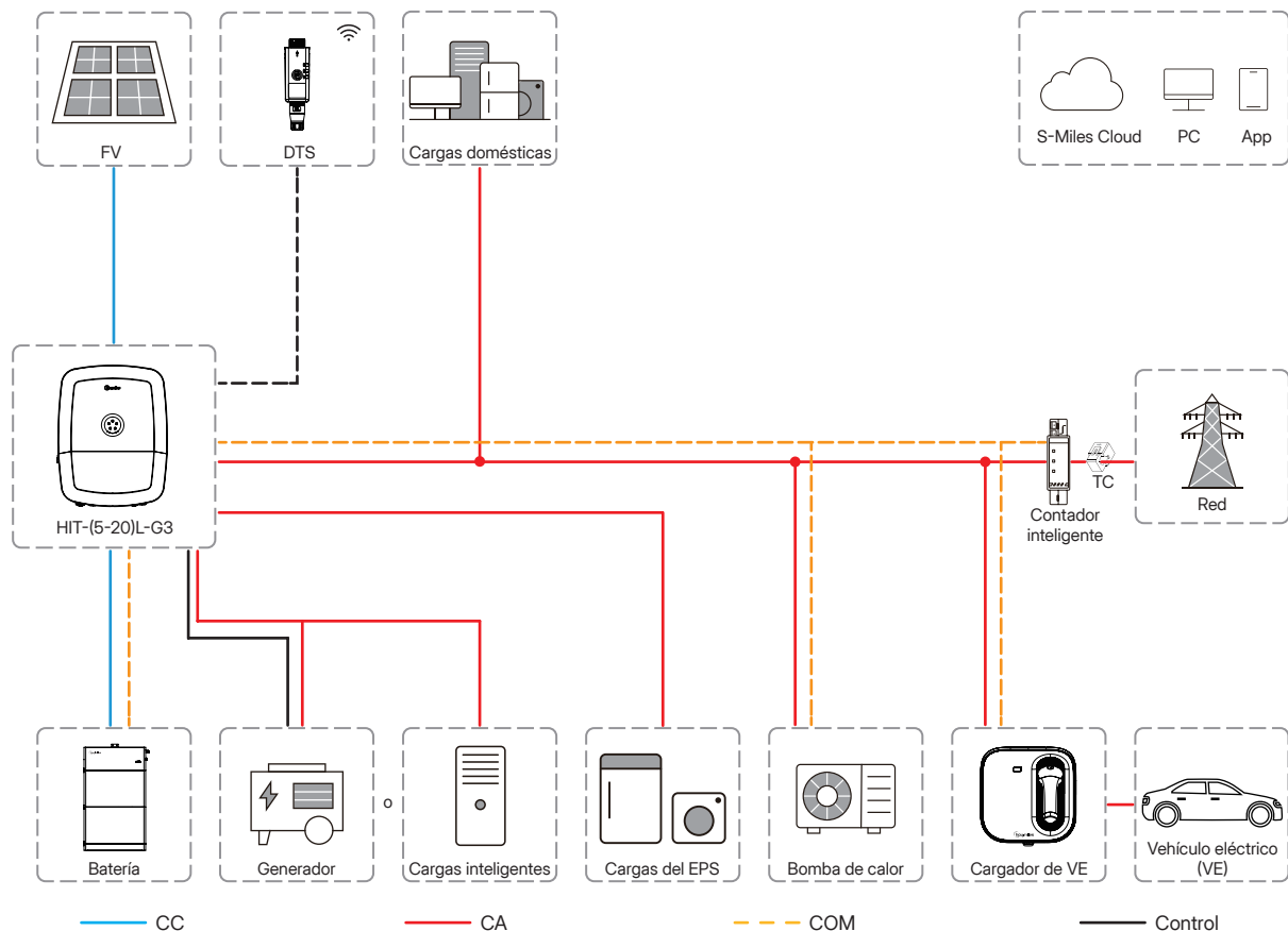
Figura 5-1 Sistema básico
