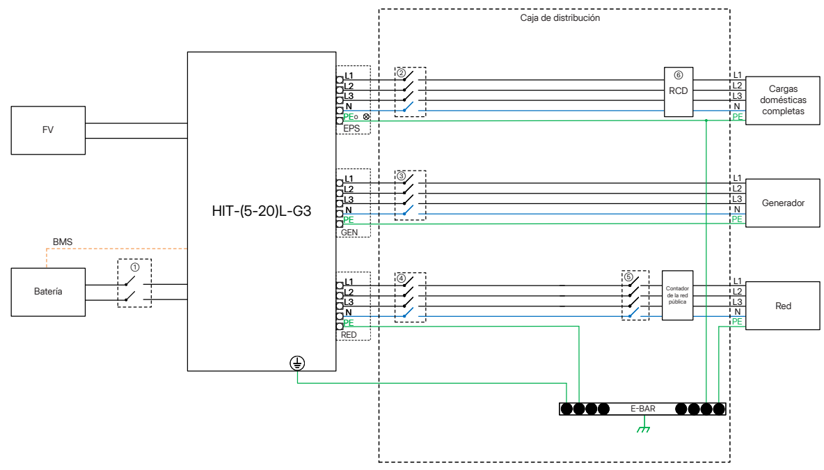
Figura 7-2 Diagrama de las cargas domésticas completas
