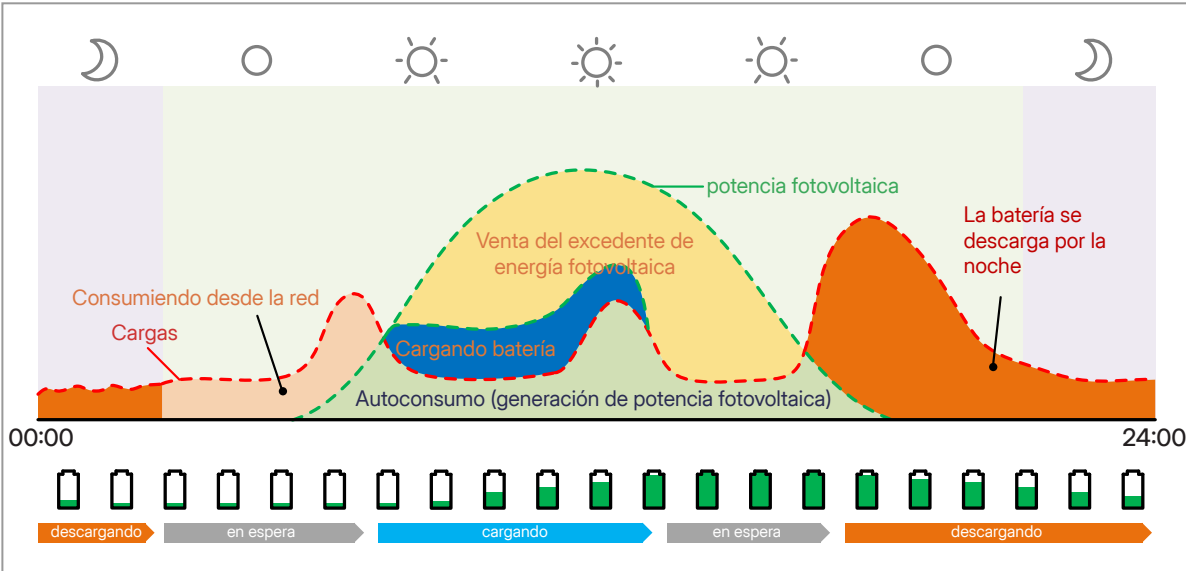
Figura 4-8 Flujo de energía del modo de autoconsumo
