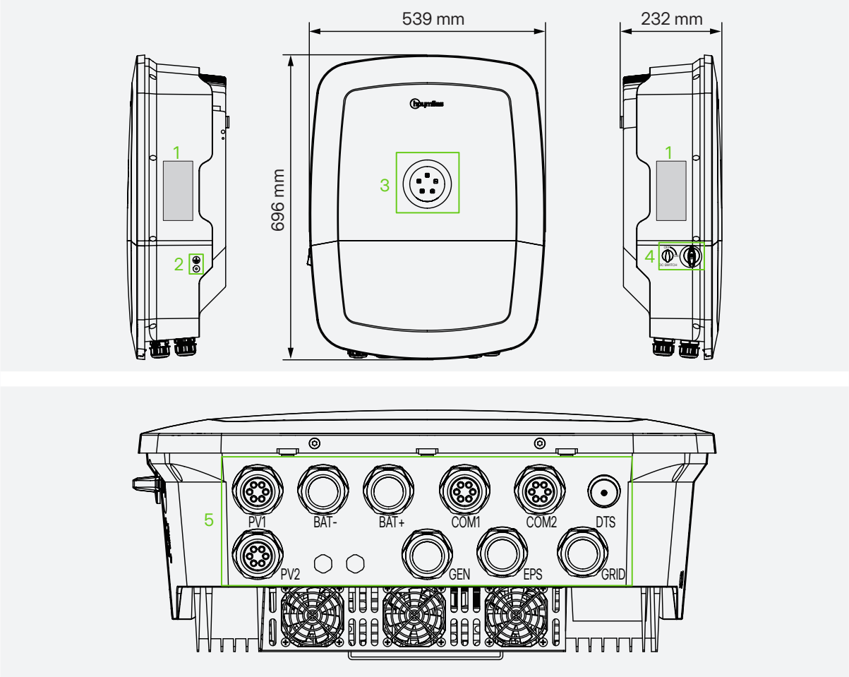
Figura 4-1 Aspecto y dimensiones
