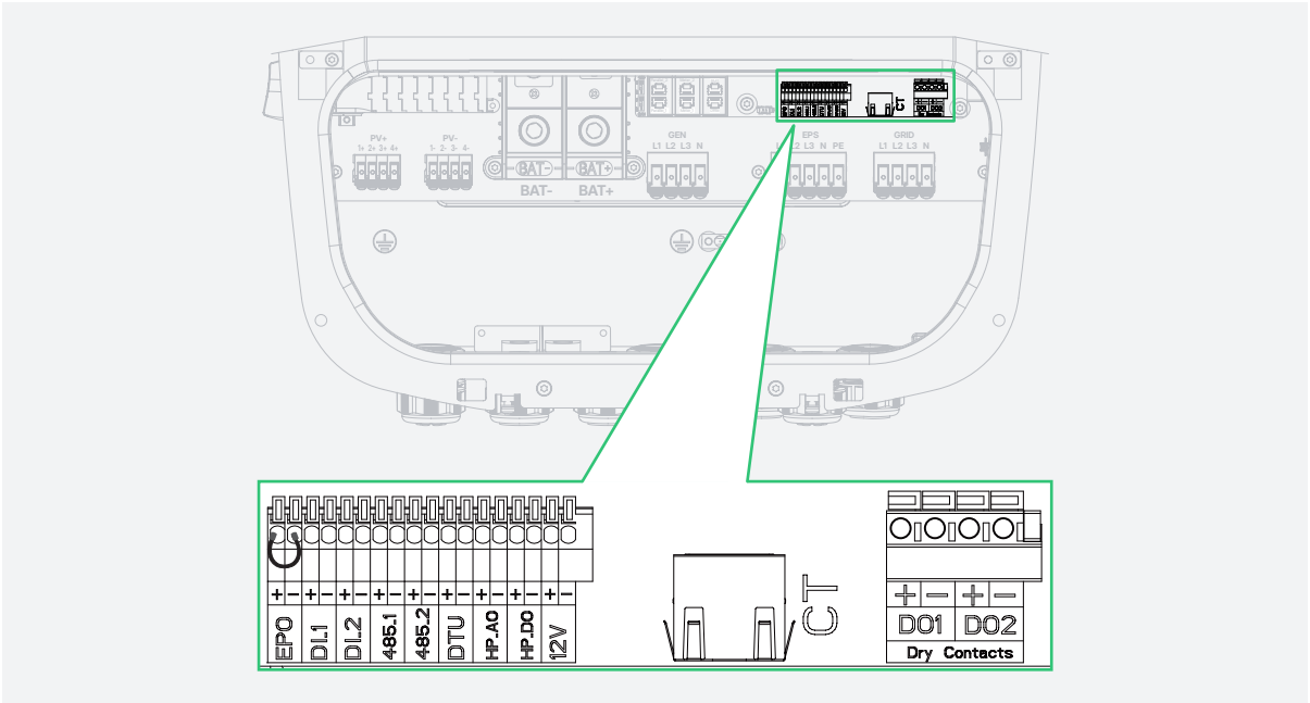
Figura 7-10 Vista general de COM2
